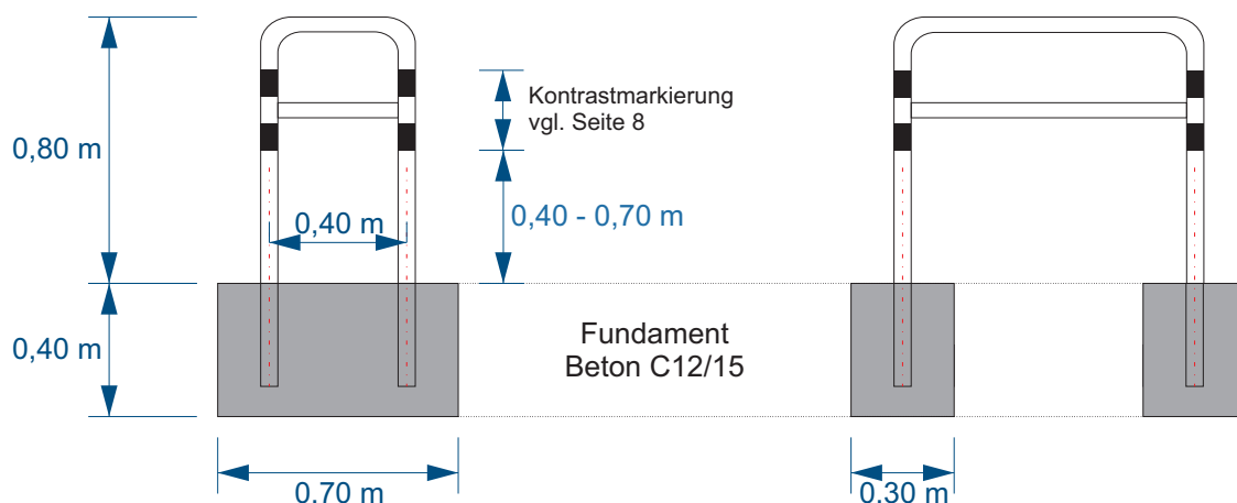
Abbildung 9: Gestaltung von Fahrradanhängerbügel mit Wechselkontrast
