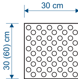
Noppenplatte
