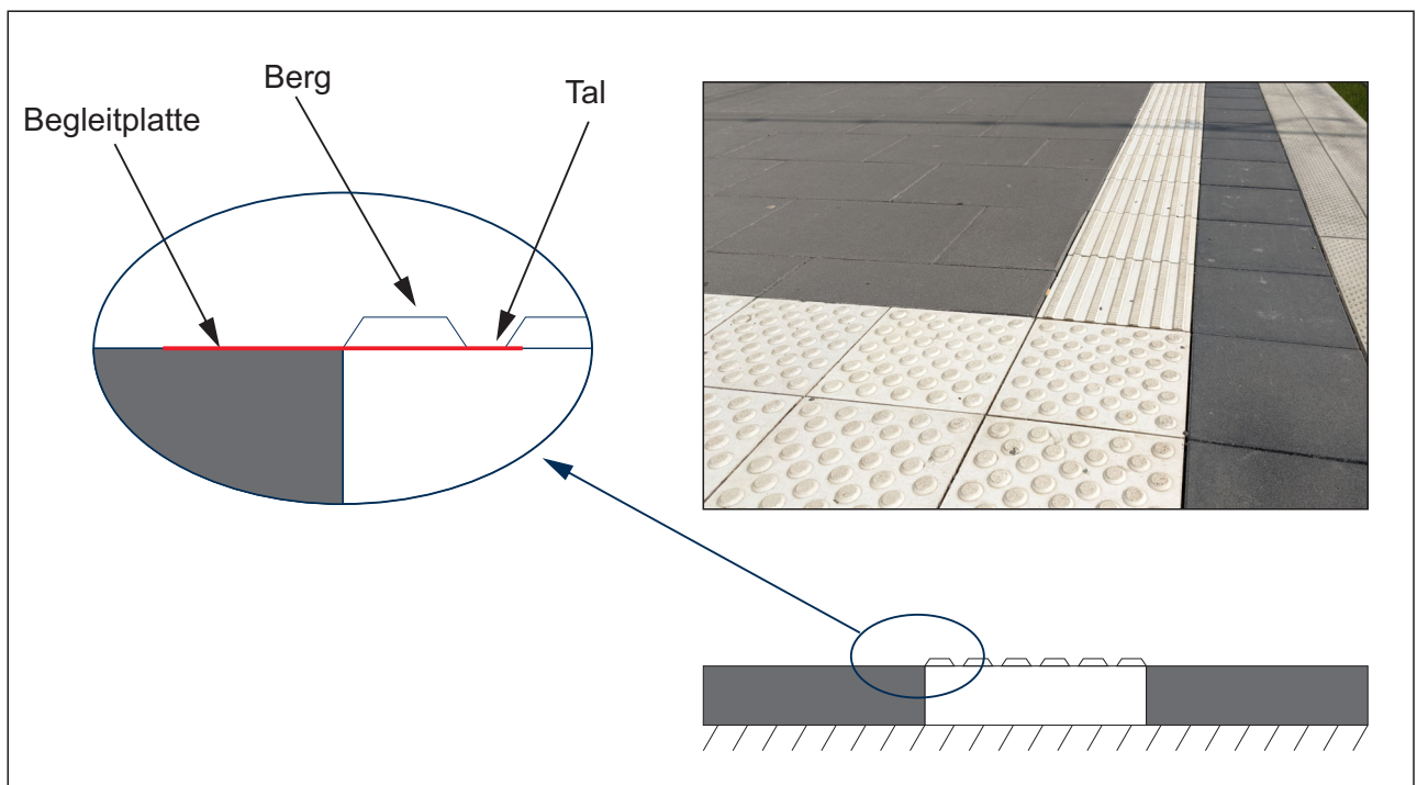
Abbildung 10: Talbündigkeit von Bodenindikatoren
