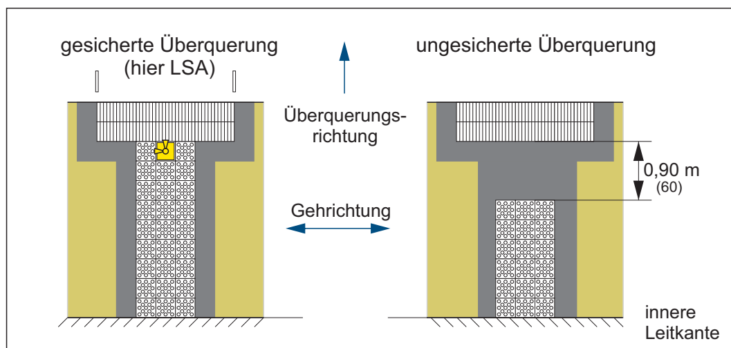
Abbildung 14: Unterscheidung gesicherte und ungesicherte Überquerungsstelle
