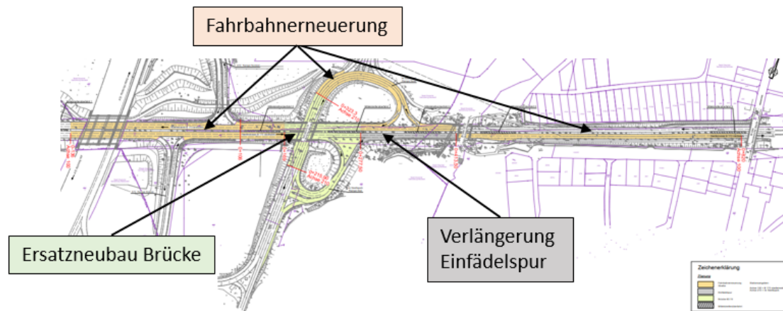
Erneuerung aller Asphaltschichten auf 1200 m Länge, Einsatz von lärminderndem Asphalt
