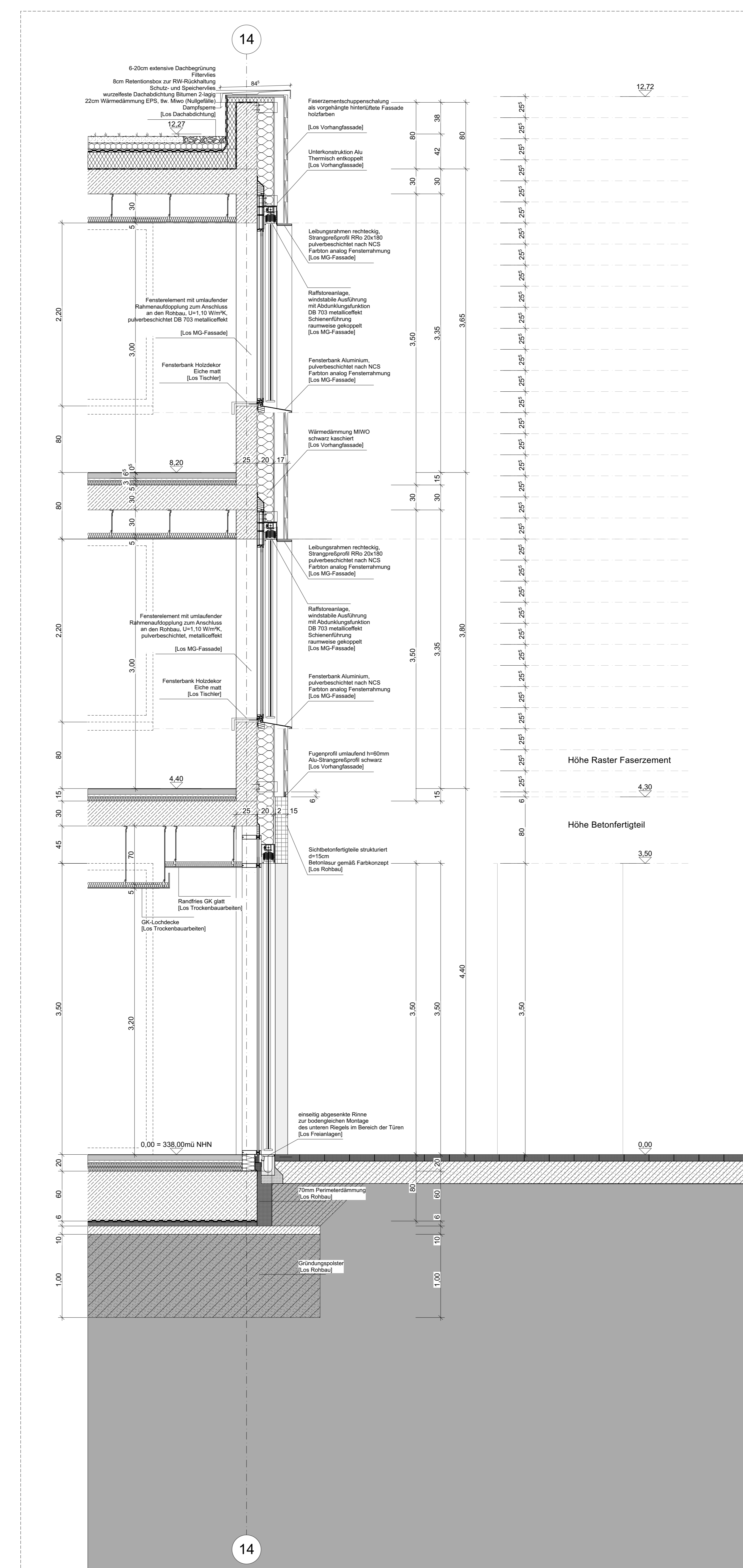
FASSADENSCHNITT SCHULE ACHSE 14 - NORDSEITE
